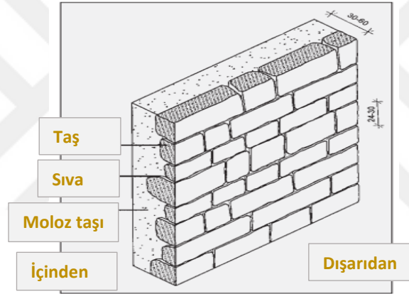
Şekil 3.12 Taş kaplı Duvarın Dışarıdan Üçlü Görünümü (Abuarkub, 2017)
