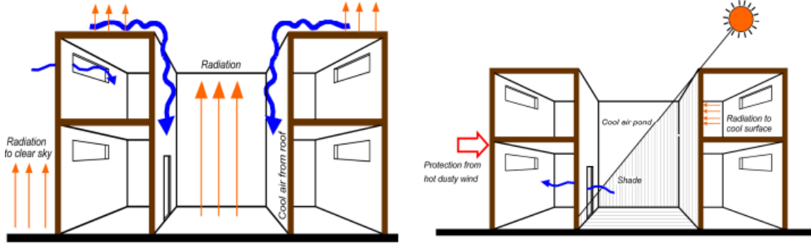
Şekil 3.10 İç Avlunun Gündüz ve Gece Termal Performansı (Muheisen, 2009)
